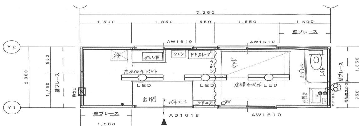
平面図 S=1/50
